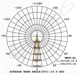
配光曲线
