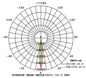
配光曲线
