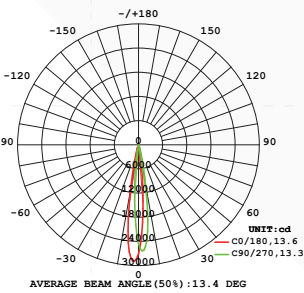
配光曲线
