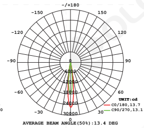
配光曲线
