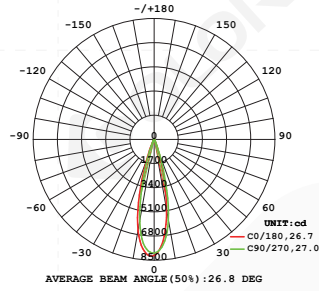
配光曲线
