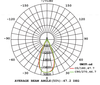
配光曲线
