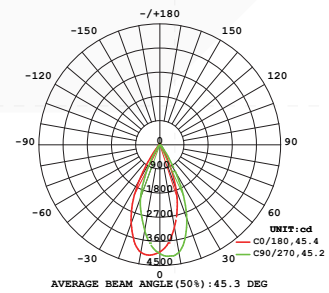
配光曲线
