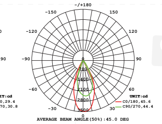
配光曲线
